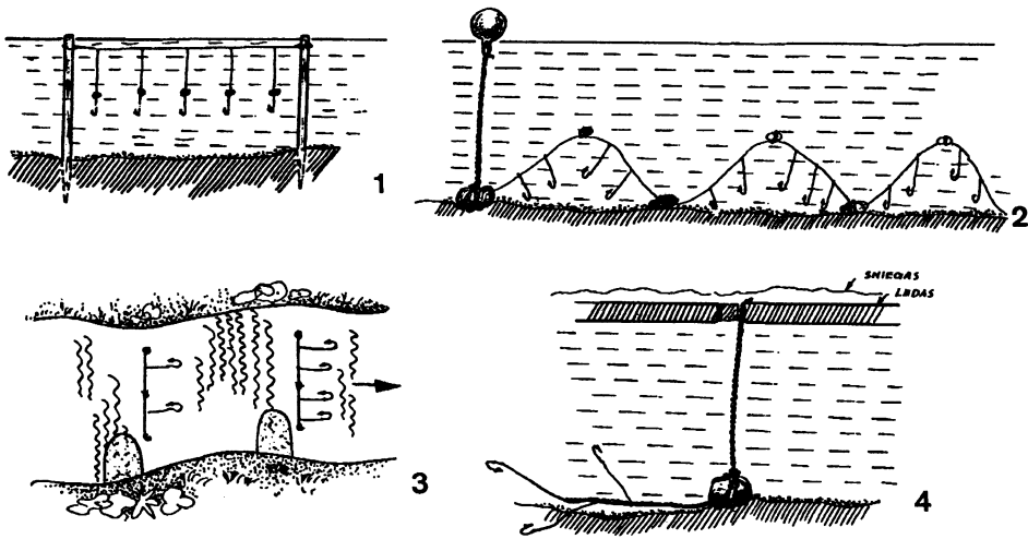
2 pav. Metinių statymo būdai: 1 – lydekoms gaudyti Mituvos ežere (Kupiškio r.), 2 – lydekoms gaudyti Vištyčio ežere, 3 – Nemune netoli Jurbarko, 4 – Nemune ties Prienais žiemą. Pagal žvejų pasakojimus 1994 m. rekonstravo R. Butvilienė
