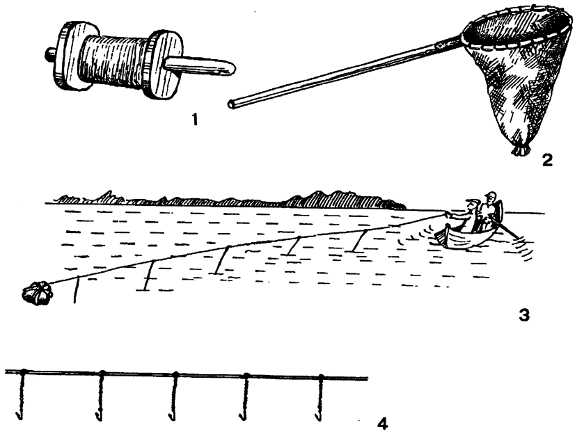
10 pav. 1 – Ritė vieliniam metiniui, 2 – graibštelis žuvims semti, 3 – metinio metimas, 4 – vielinis metinys su pavadėliais. Pagal žvejų pasakojimus 1992 m. rekonstravo R. Butvilienė
