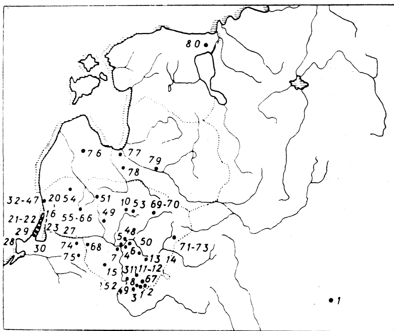
4 pav. Rytų Pabaltijo vienasluoksniai virvelinės keramikos kultūros paminklai:
