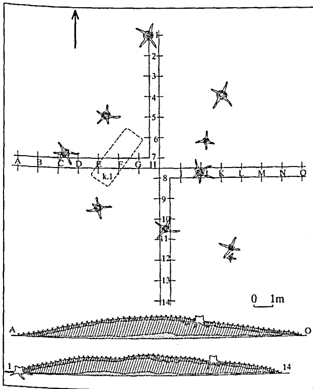
3 pav. Pilkapis Nr. I planas.
