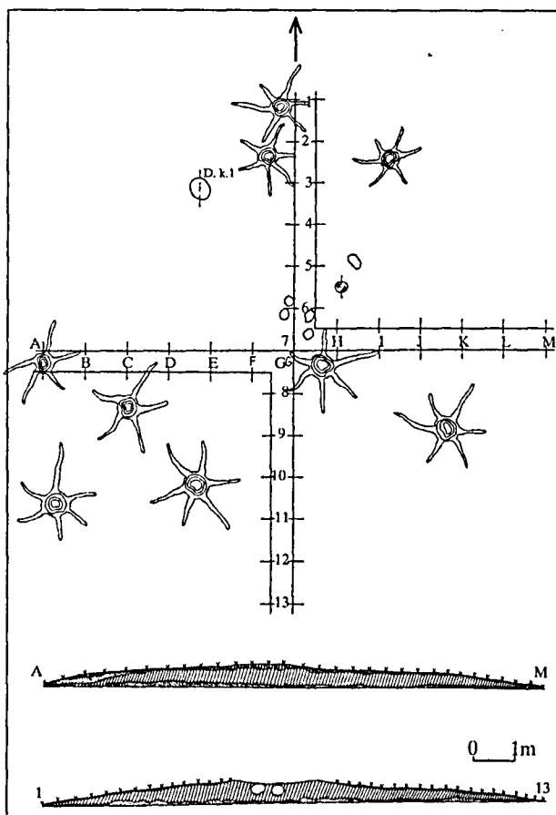
14 pav. Pilkapio Nr. VII planas.
