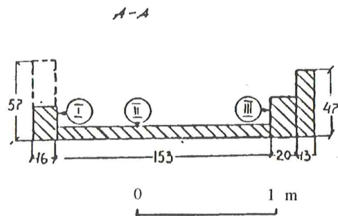
8 p a v. IV krosnies pakuros liekanos, planas ir pjūvis A-A: 1 – pakuros sienelės, 2 – padas, 3 – perdangos atramos. Piešė Verutė Trečiokienė.
