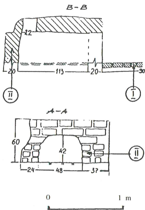
6 p a v. III krosnies planas ir pjūviai (B-B, A-A): I – aikštelė prie pakuros, II – pakura. Piešė Verutė Trečiokienė.
