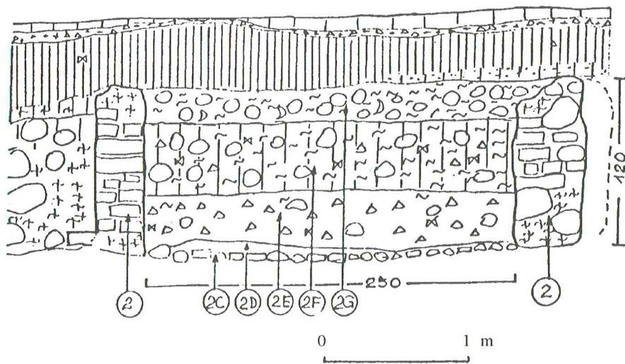
12 p a v. VI krosnies pjūvis: 2 – pakuros sienelės, 2C – plytų padas, 2D – pelenai, 2E – plytų nuolaužos, akmenys, 2F – akmenys, molis, juodžemis, 2G – molis, keramika, akmenys. Piešė Verutė Trečiokienė.
