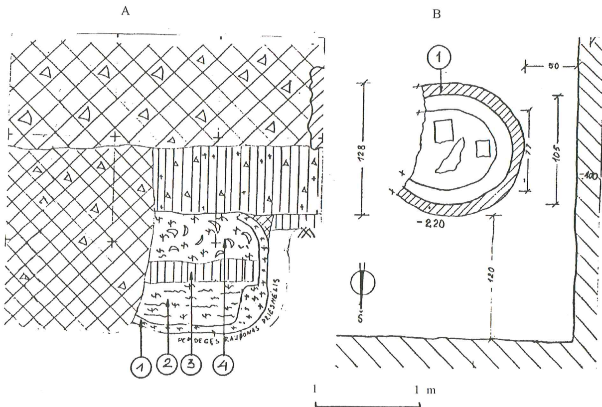
4 p a v. II krosnies pjūvis (A) ir planas (B): 1 – molinis padas ir sienelės, 2 – pelenai su degto molio gabalais, 3 – juodžemis su degėsiiais, 4 – degto molio gabalai su keramikos šukėmis. Piešė Verutė Trečiokienė.
