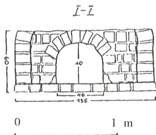
10 p a v. V krosnies planas ir pjūviai (I-II): 1 – pakuros sienelės, 2 – plytų padas, 3 – skliautas-dūmtraukis, 4 – kamino pamatas, 4a – molio juosta. Piešė Verutė Trečiokienė.
