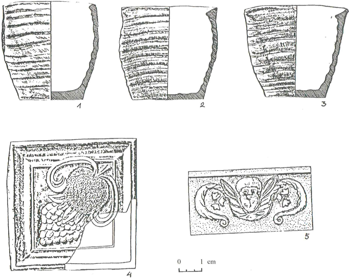
11 p a v. Keramika iš V krosnies: 1, 2, 3 – puodyniniai kokliai su kvadratine anga, 4 – plokštinis koklis, 5 – karnizinis koklis. Piešė Verutė Trečiokienė.
