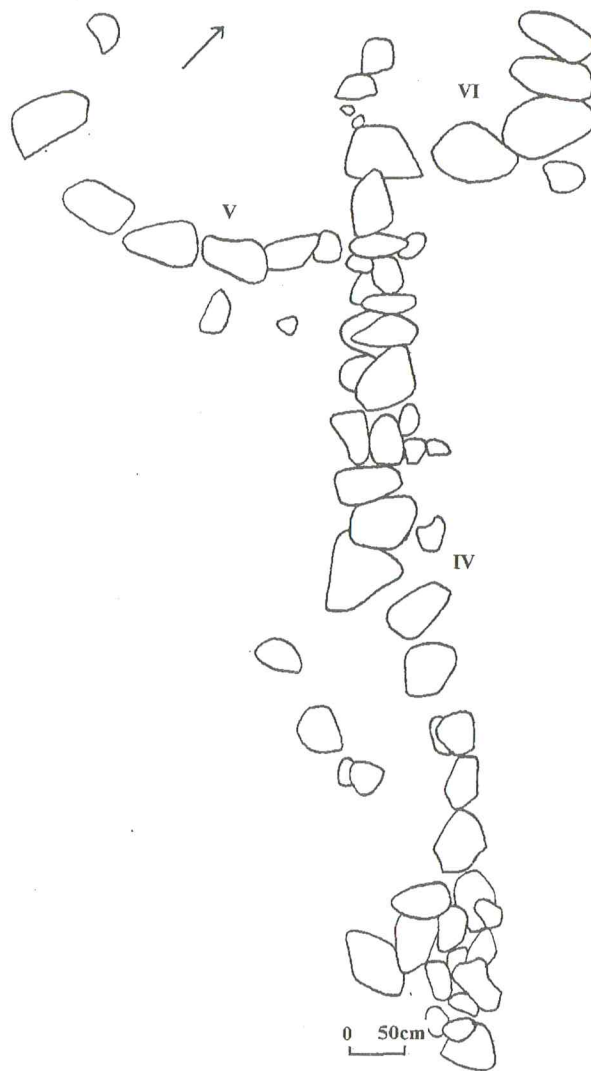
26 pav. IV, V ir VI akmenų vainikai. Piešė I. Keršulytė
